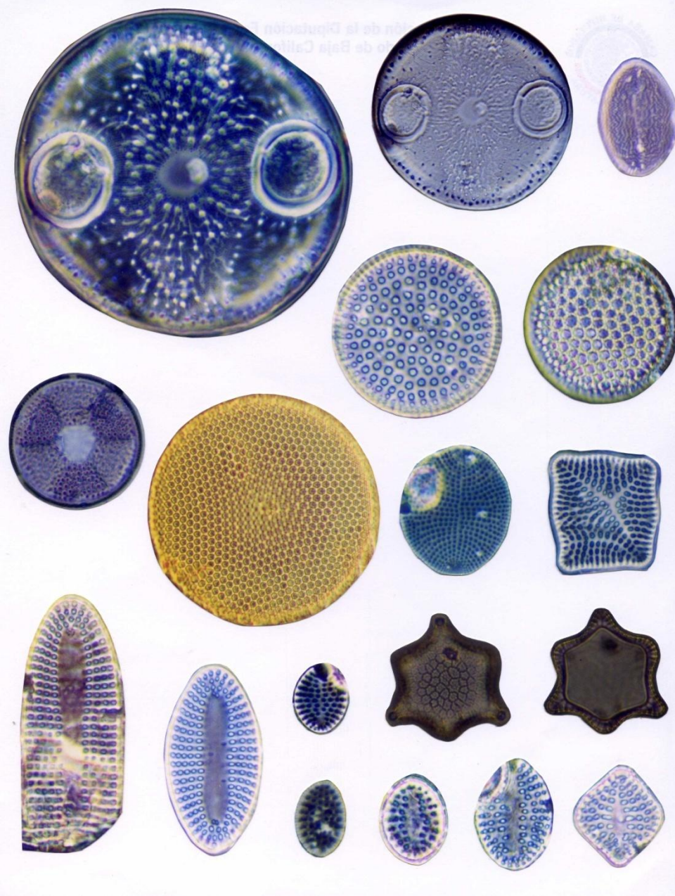
DIATOMEAS BENTÓNICAS
